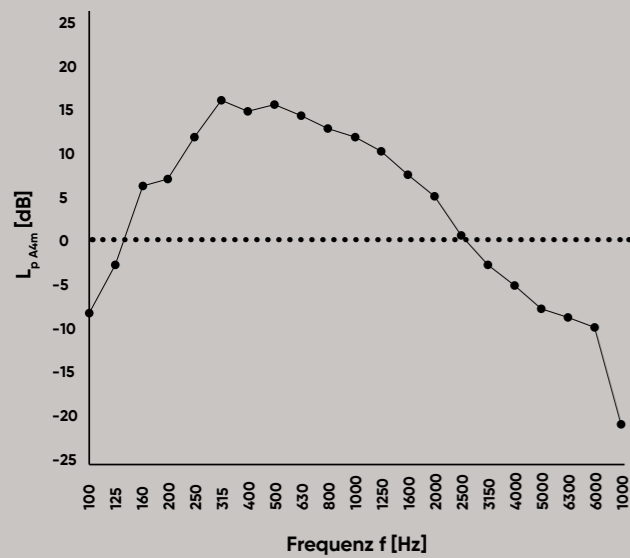
Schallpegel der Lüftung außerhalb der Schallschutzkabine
