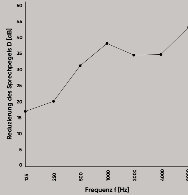
Verringerung des Sprechpegels
