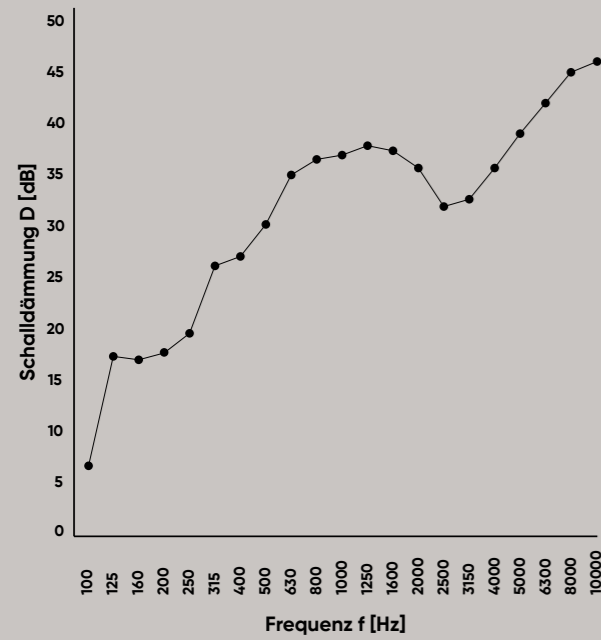
Der gewogene Schalldämmungskoeffizient
