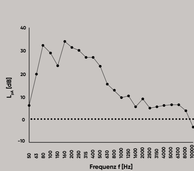
Schallpegel der Lüftung innen der Schallschutzkabine
